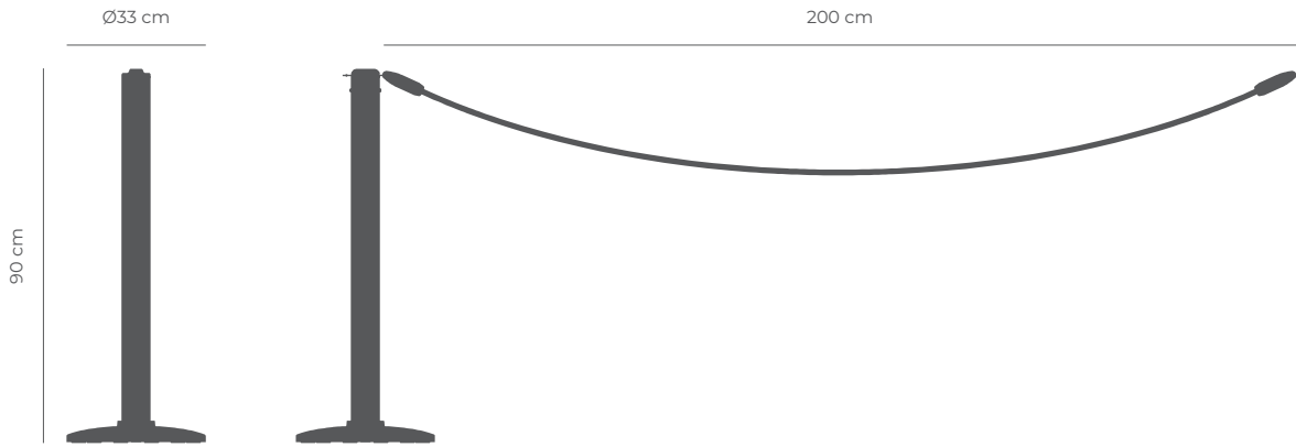
Versátil + Gancho Abierto Esc. 1:20 (Peso: 8kg)
