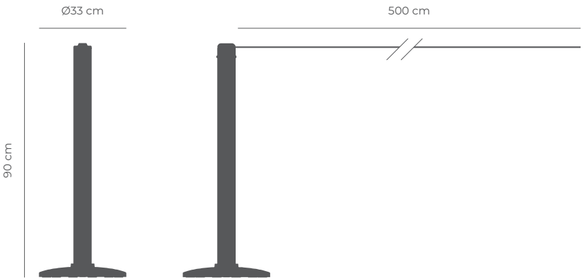
Versátil + Prensa Gomas Esc. 1:20 (Peso: 8kg)
