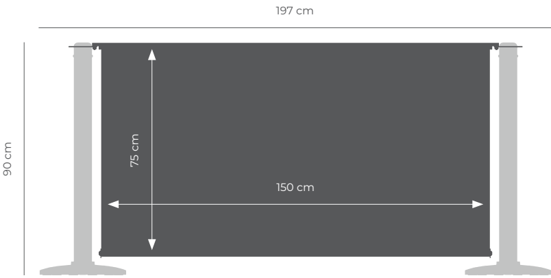
Banner Esc. 1:20 (Peso: 20kg)
