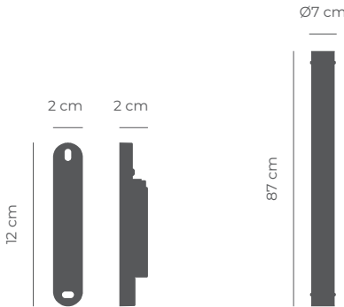
Terminal mural Esc. 1:5 (Peso: 0,01kg) Tubo Auxiliar Esc. 1:20 (Peso: 1kg)
