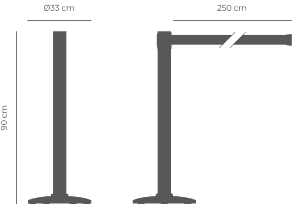
Retr  ctil Esc. 1:20 (Peso: 8kg)
