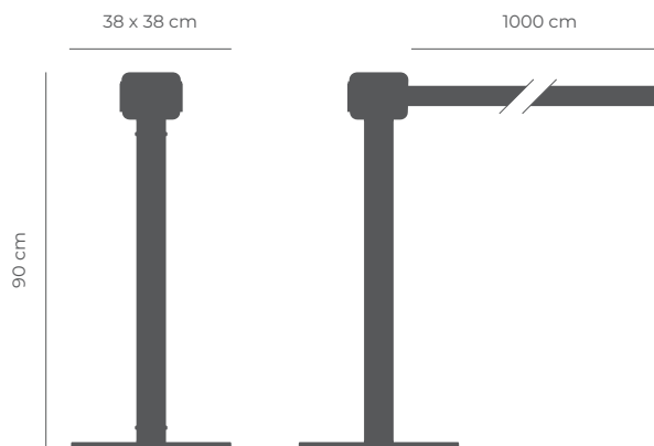
BASIC Esc. 1:20 (Peso: 10kg)
