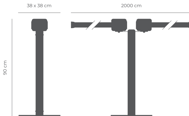
DOUBLE Esc. 1:20 (Peso: 11,35kg)
