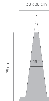
Cono recomendado(*) Esc. 1:20 (Peso: 6kg)
